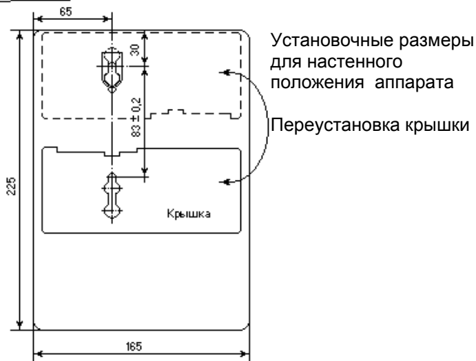
Рисунок 2.1 - Вид аппарата снизу
