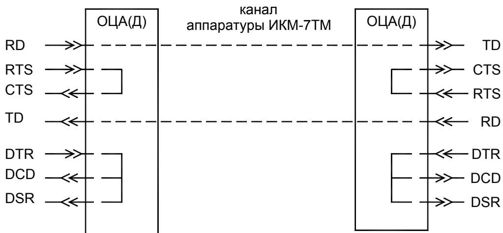
Рисунок 5 – «Непрозрачный» режим канала RS-232
