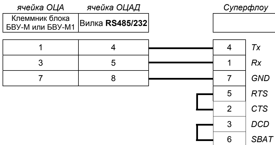
Рисунок 9 – Схема подключения к барьеру ISCOM
