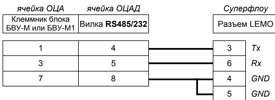
Рисунок 8 – Схема подключения к вычислителю «Суперфлюу-II»
