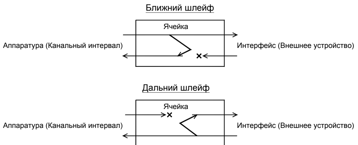
Рисунок 6 – Понятие «ближнего» и «дального» шлейфов
