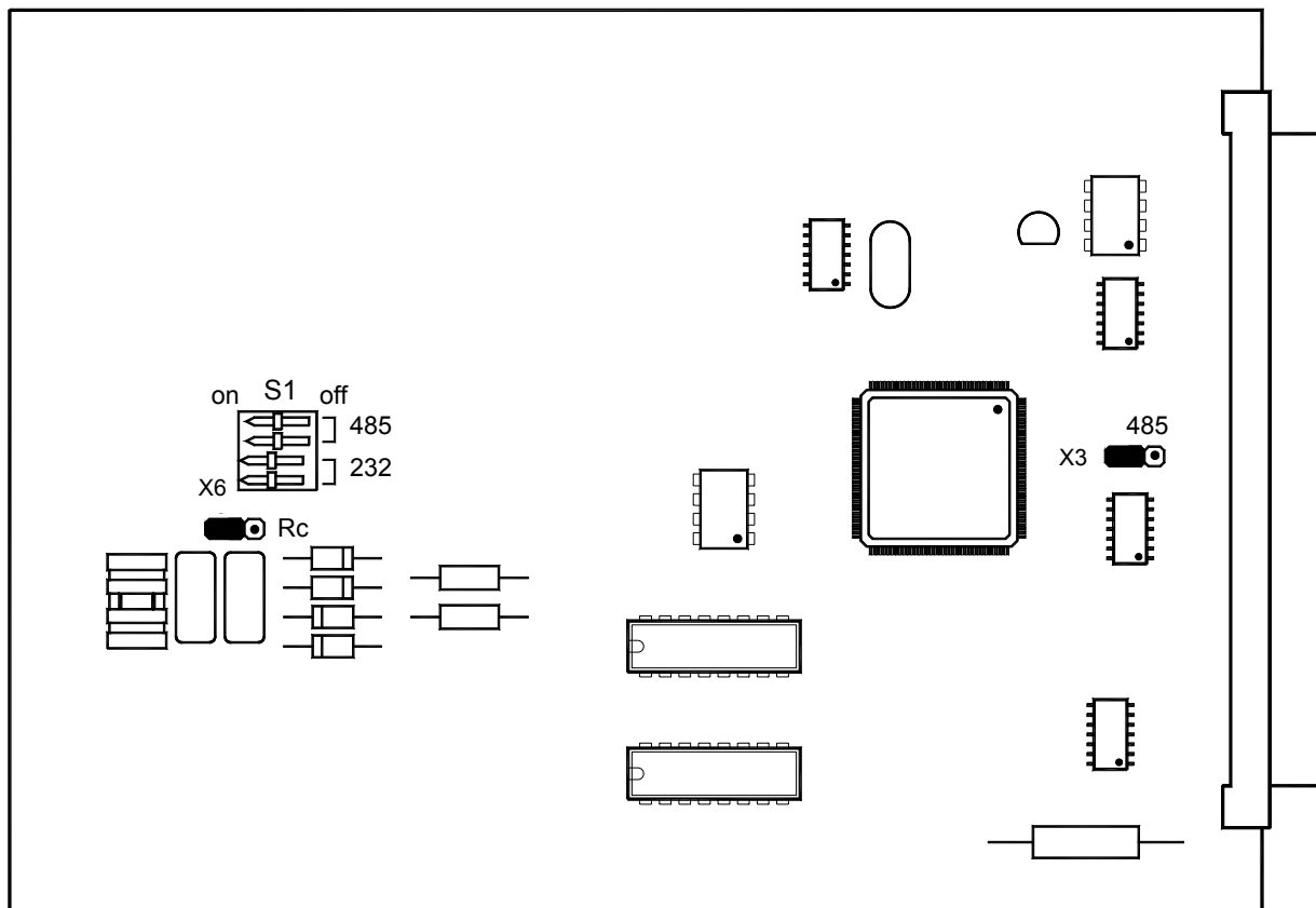
Рисунок 1 – Расположение джамперов и переключателя в ячейке ОЦА/ОЦАД (переключатель S1 устанавливается только в ячейке ОЦА)
