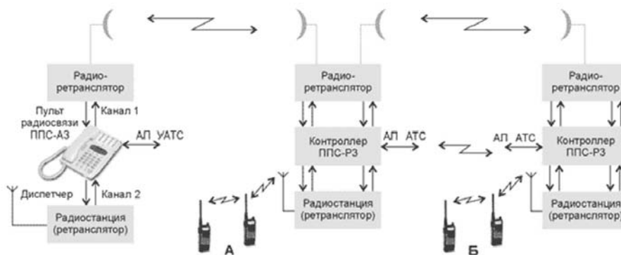
Рисунок 4.7 – Организация системы радиосвязи по радиорелейной линии
